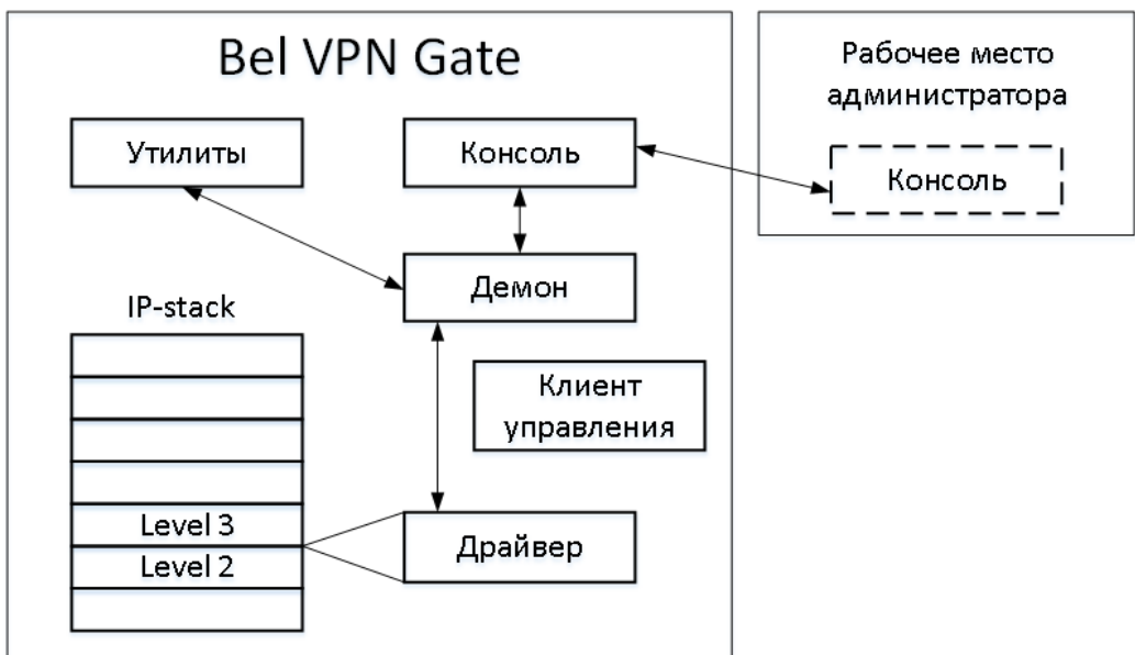
Рисунок 2 Схема взаимодействия модулей
